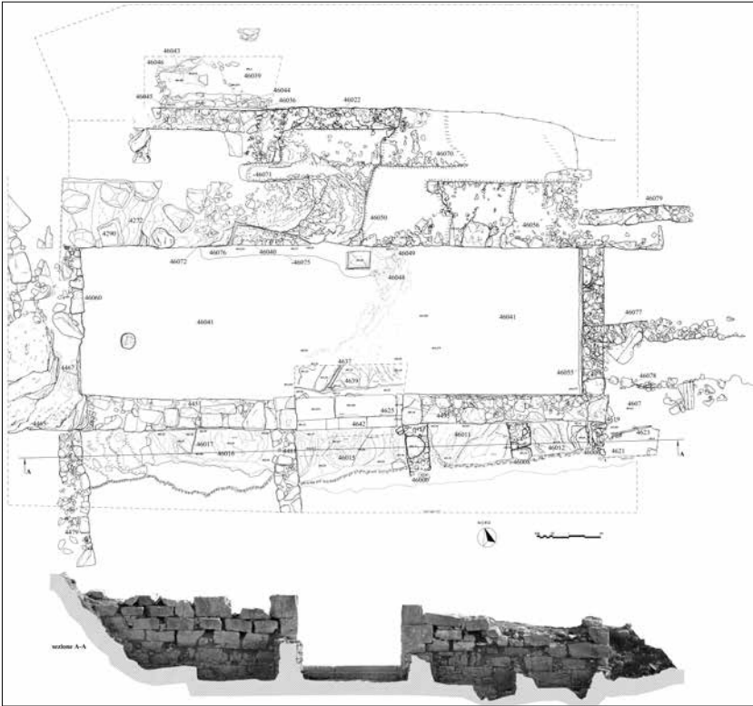
4. Segesta. Ephibikon . Pianta (2023) e modello 3D del prospetto (C. Cassanelli).
